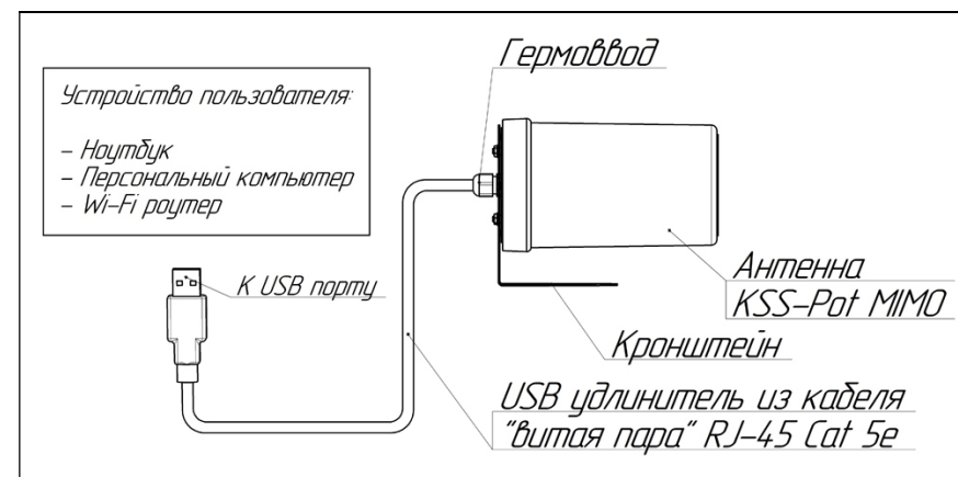
Схема 2 – Подключение комплекта к пользовательскому устройству
